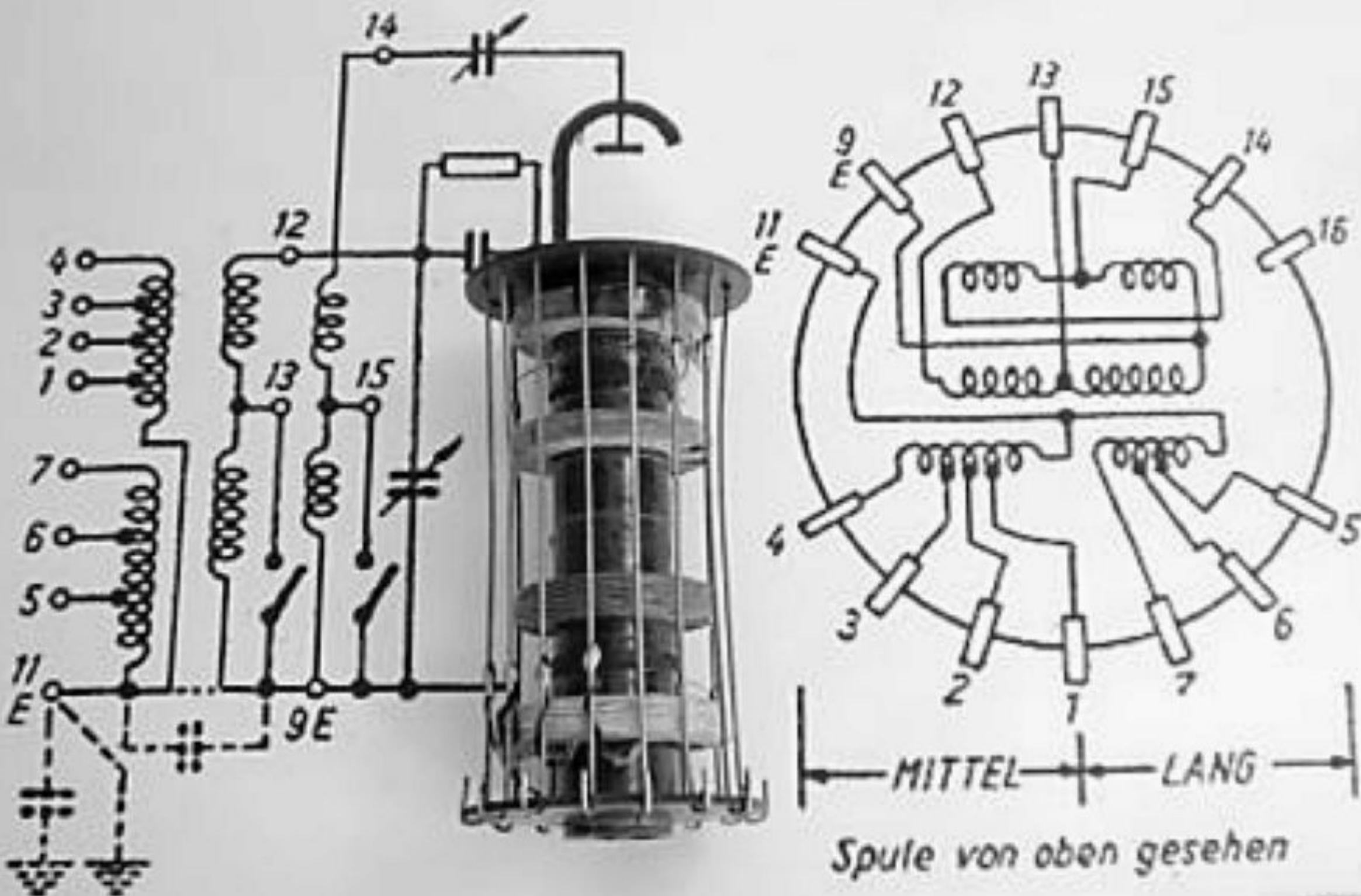
Spulenanschlüsse des VE 301 (Käfigspule)
